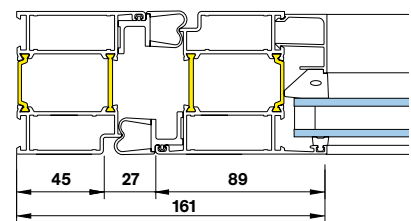
Klemfri bakkant med smal- eller modulprofil
