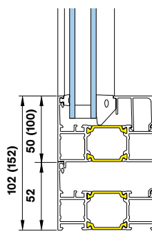
Fast sideparti med alt. påbyggingsprofiler
