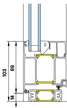
Isolert terskel med anslagsdør
