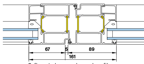
2-fløyet dør med smalprofil
