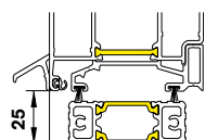
Isolert terskel med børstetettinger i uk. dør
