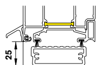
Uisolert terskel med børstetettinger i uk. dør
