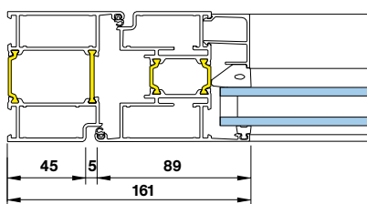
Smalprofil for Fixbeslag
