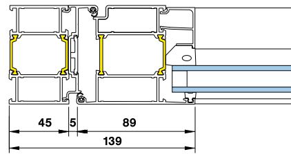
Smalprofil med utskiftbare anslag
