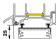
Rustfri uisolert terskel med børstetettinger i uk. dør
