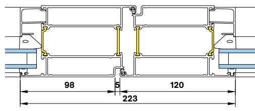
2-fløyet dør med modulprofil
