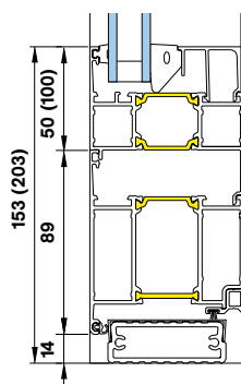
Rustfri uisolert terskel med anslagsdør
