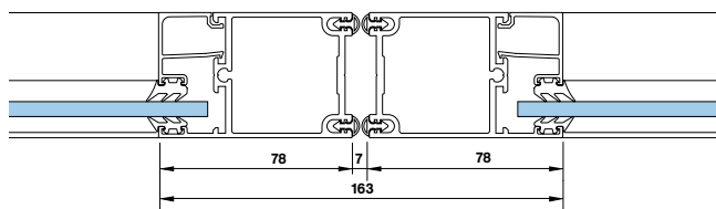
Dobbelt dører uten anslag, smalprofil
