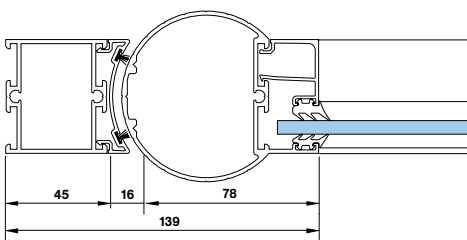
Klemfri bakkant, avrundet aluminiumprofil
