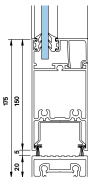
Sokkelprofil med børstetetting
