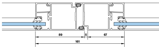
Møtegående dører, smalprofil
