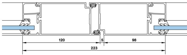
Møtegående dører, modulprofil
