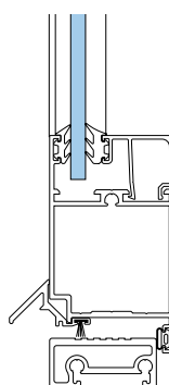
Helgjærede dørblad, innadslående med anslagstetting
