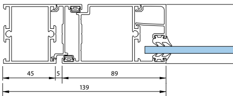
Smalprofil med utskiftbart anslag
