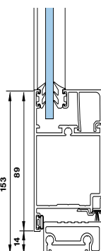
Helgjærede dørblad, utadslående med anslagstetting
